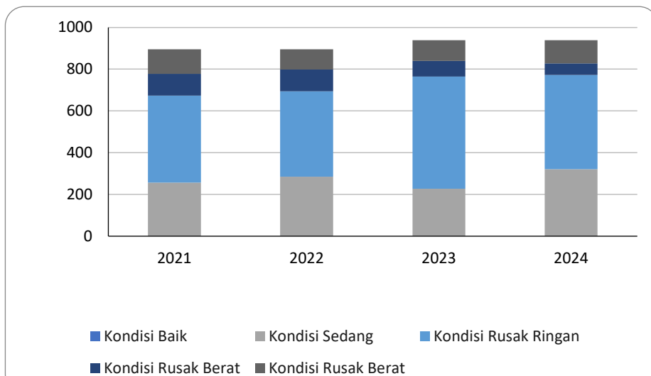
Grafik. 4.2.2 Panjang Jalan Provinsi menurut Kondisinya (km) di Provinsi Kalimantan Timur, 2021-2024
