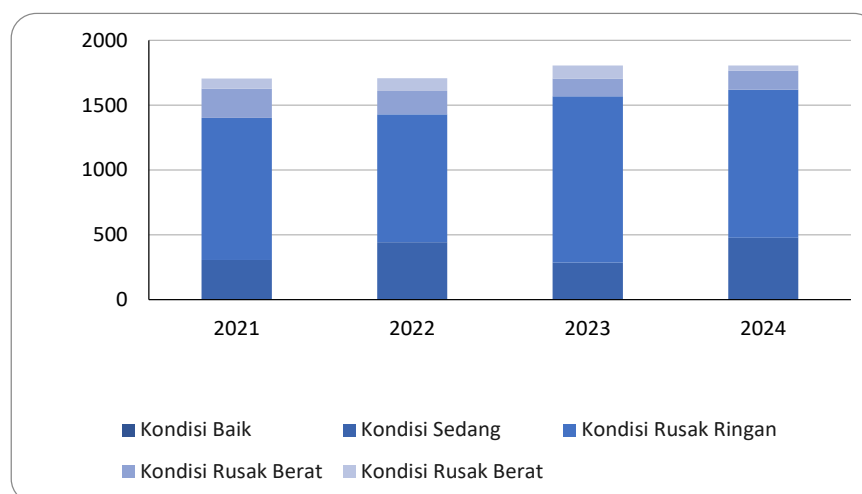
Grafik. 4.2.1 Panjang Jalan Nasional di Provinsi Kalimantan Timur menurut Kondisinya (km), 2021-2024
